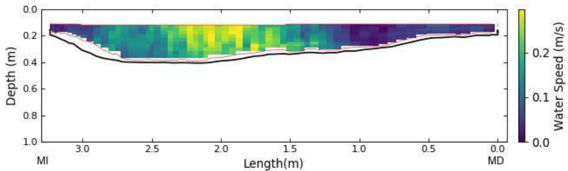
Figura A.75. Distribución de velocidades en la sección de aforo de la EM41 obtenida con ADCP. En el gráfico se señala la ubicación de la margen izquierda (MI) y de la margen derecha (MD).
