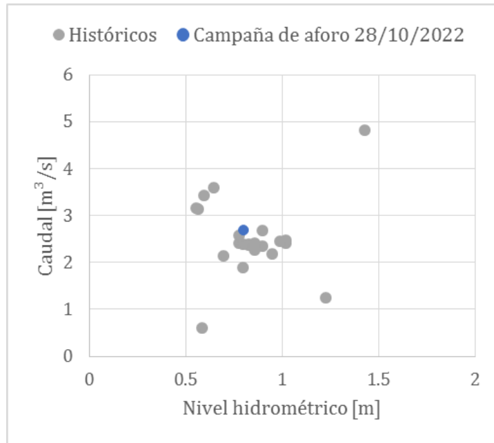
Figura A.35. Registros históricos de niveles y caudales en la EM13.
