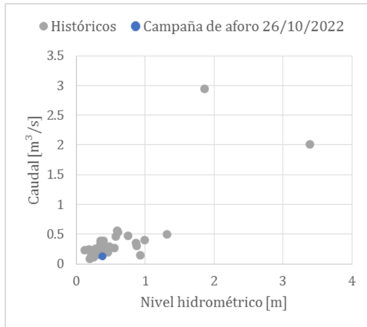
Figura A.87. Registros históricos de niveles y caudales en la EM72.
