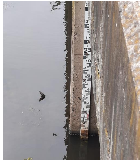
Figura A.16. Precipitaciones en la cuenca en la semana previa al aforo (izquierda) y nivel del curso registrado por la regla hidrométrica (derecha).
