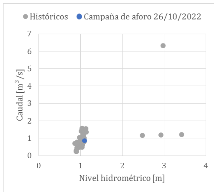
Figura A.24. Registros históricos de niveles y caudales en la EM11.
