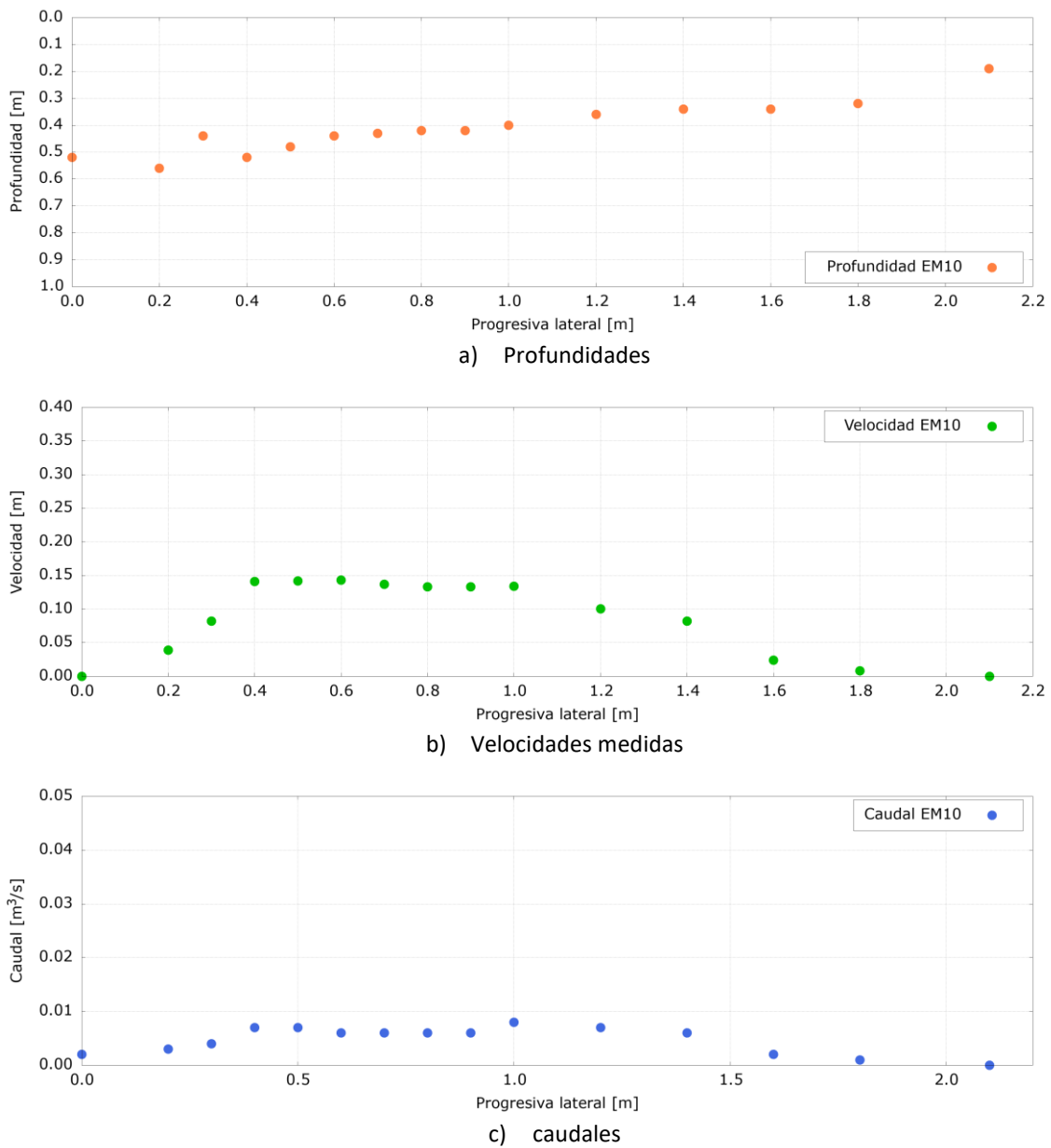
Figura A.18. Distribución de profundidades, velocidades medidas y caudales en la sección de aforo de la EM10 obtenida con ADV. La progresiva lateral 0 se corresponde con la margen izquierda.
