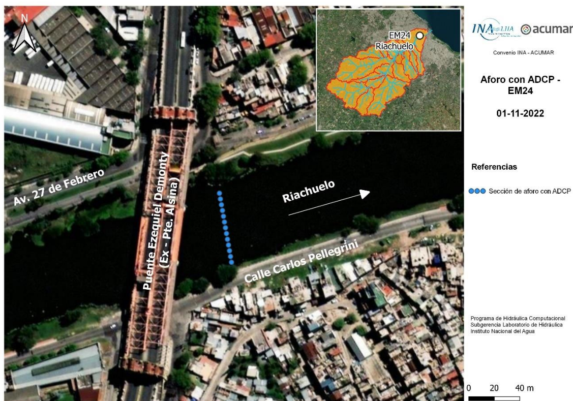
Figura A.60. Sección de aforo en la EM24.
