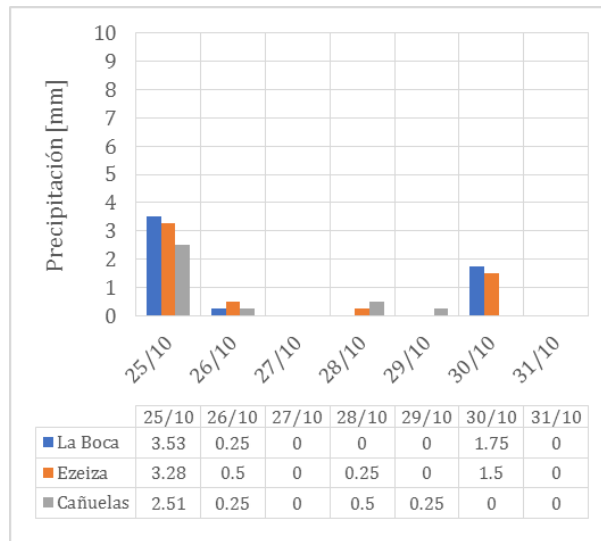
Figura A.67. Precipitaciones en la cuenca en la semana previa al aforo en la EM30.
