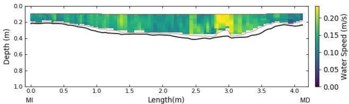
Figura A.86. Distribución de velocidades en la sección de aforo de la EM72 obtenida con ADCP. En el gráfico se señala la ubicación de la margen izquierda (MI) y de la margen derecha (MD).
