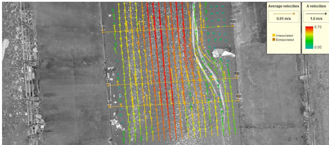
Figura A.95. Campo de velocidades superficiales en la EM76 obtenido con el software Fudaa.
