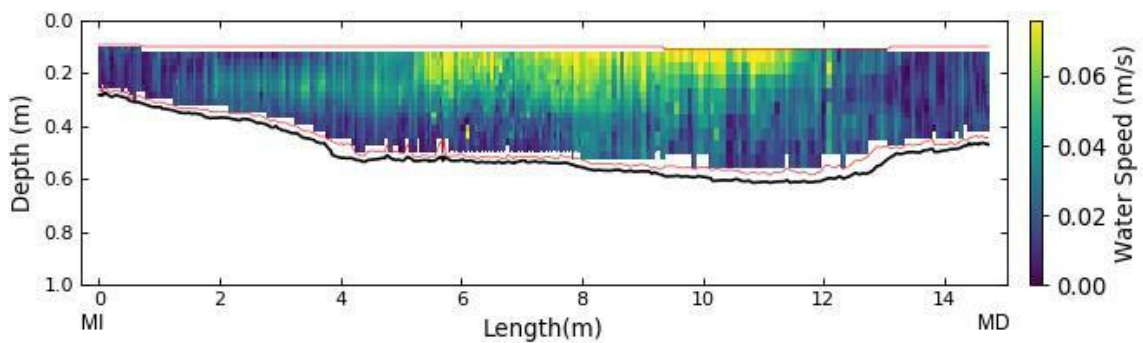
Figura A.91. Distribución de velocidades en la sección de aforo de la EM73 obtenida con ADCP. En el gráfico se señala la ubicación de la margen izquierda (MI) y de la margen derecha (MD).
