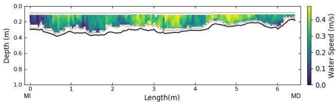
Figura A.39. Distribución de velocidades en la sección de aforo de la EM14 obtenida con ADCP. En el gráfico se señala la ubicación de la margen izquierda (MI) y de la margen derecha (MD).
