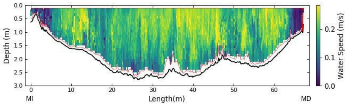
Figura A.48. Distribución de velocidades en la sección de aforo de la EM17 obtenida con ADCP. En el gráfico se señala la ubicación de la margen izquierda (MI) y de la margen derecha (MD).
