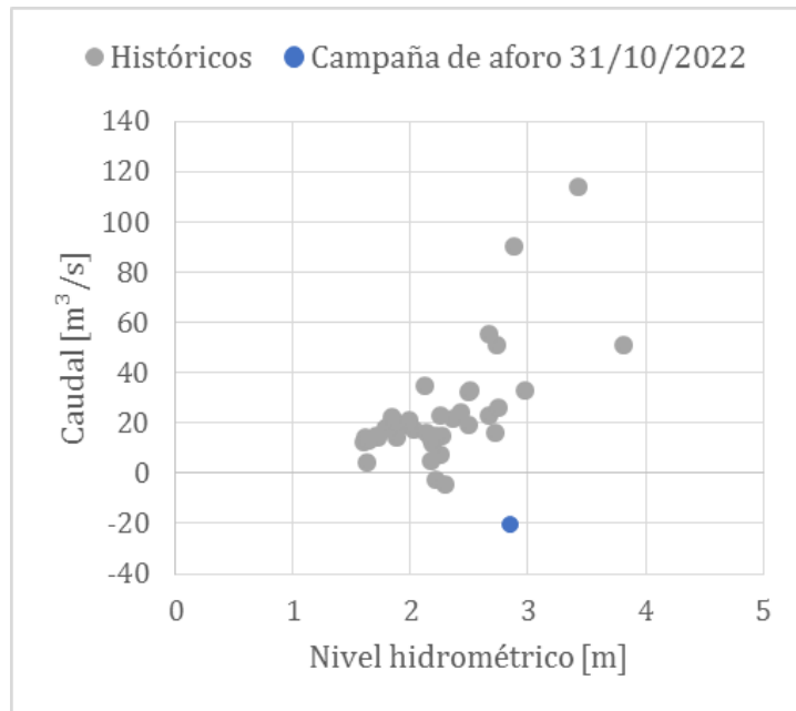
Figura A.49. Registros históricos de niveles y caudales en la EM17.
