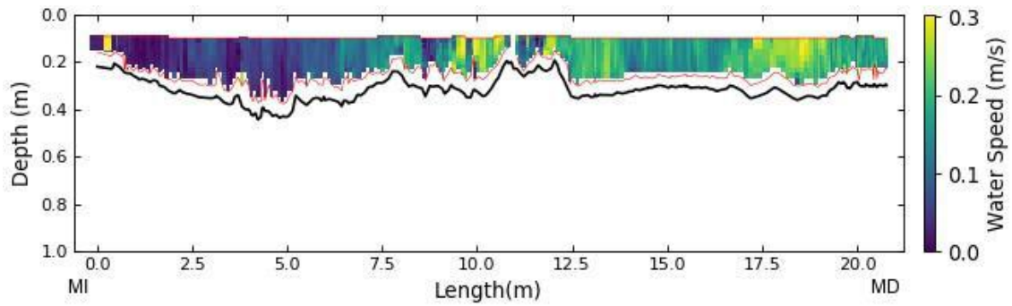
Figura A.43. Distribución de velocidades en la sección de aforo de la EM16 obtenida con ADCP. En el gráfico se señala la ubicación de la margen izquierda (MI) y de la margen derecha (MD).
