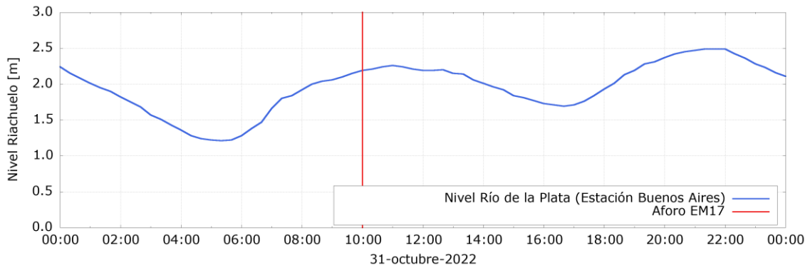
Figura A.45. Niveles registrados en la Estación Regatas de Avellaneda (ACUMAR) al momento de realizarse el aforo en la EM17.
