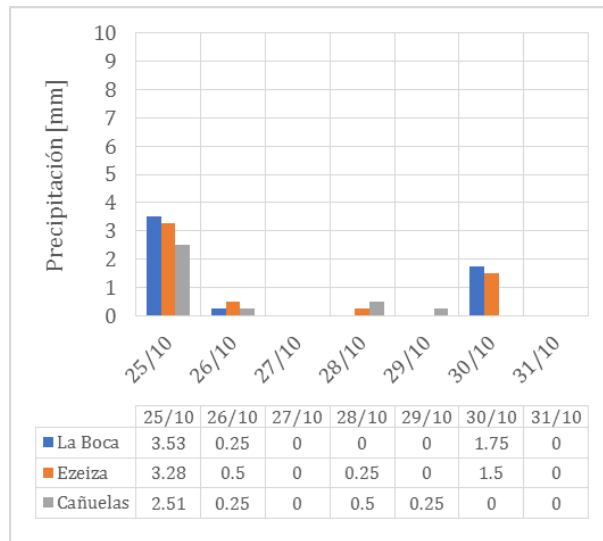
Figura A 61. Precipitaciones en la cuenca en la semana previa al aforo en la EM24.
