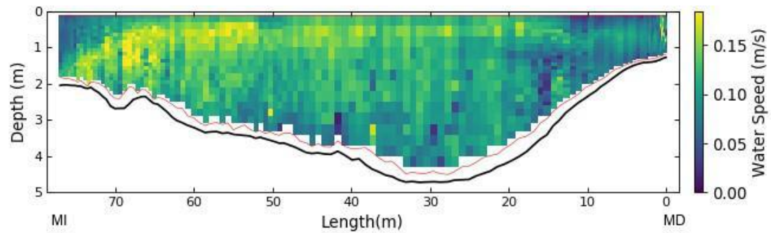
Figura A.70. Distribución de velocidades en la sección de aforo de la EM30 obtenida con ADCP. En el gráfico se señala la ubicación de la margen izquierda (MI) y de la margen derecha (MD).
