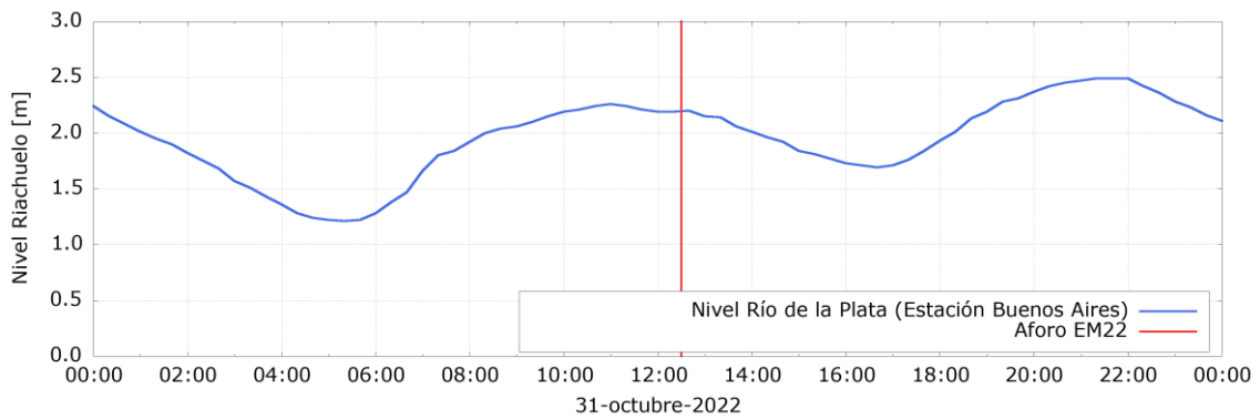
Figura A.57. Niveles registrados en la Estación Regatas de Avellaneda (ACUMAR) al momento de realizarse el aforo en la EM22.
