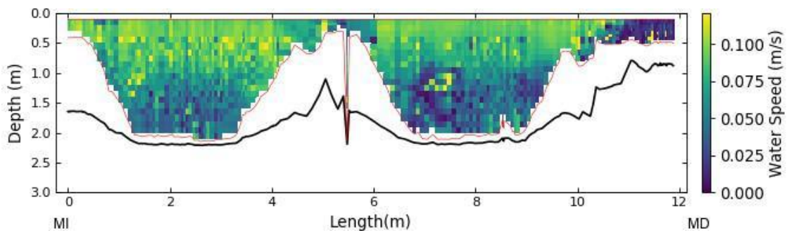
Figura A.59. Distribución de velocidades en la sección de aforo de la EM22 obtenida con ADCP. En el gráfico se señala la ubicación de la margen izquierda (MI) y de la margen derecha (MD).
