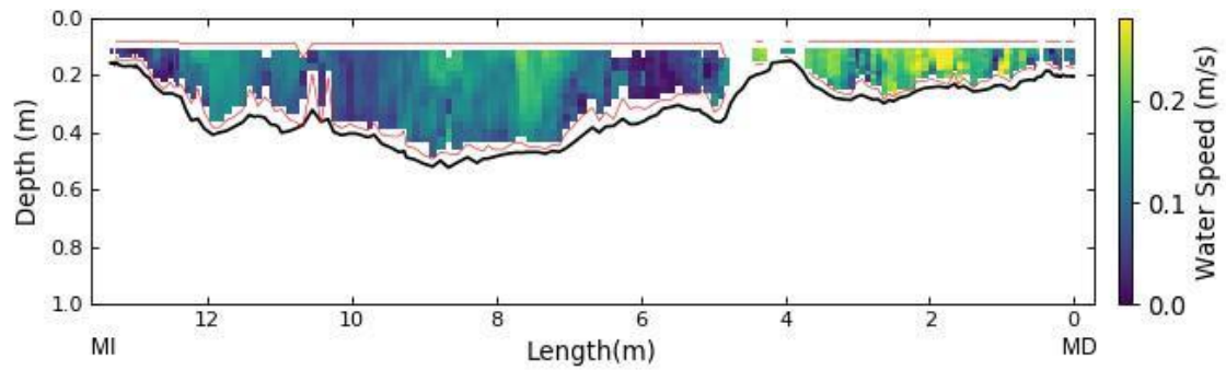
Figura A.14. Distribución de velocidades en la sección de aforo de la EM08 obtenida con ADCP. En el gráfico se señala la ubicación de la margen izquierda (MI) y de la margen derecha (MD).
