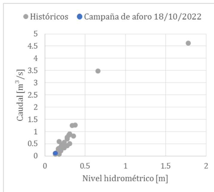
Figura A.76. Registros históricos de niveles y caudales en la EM41.
