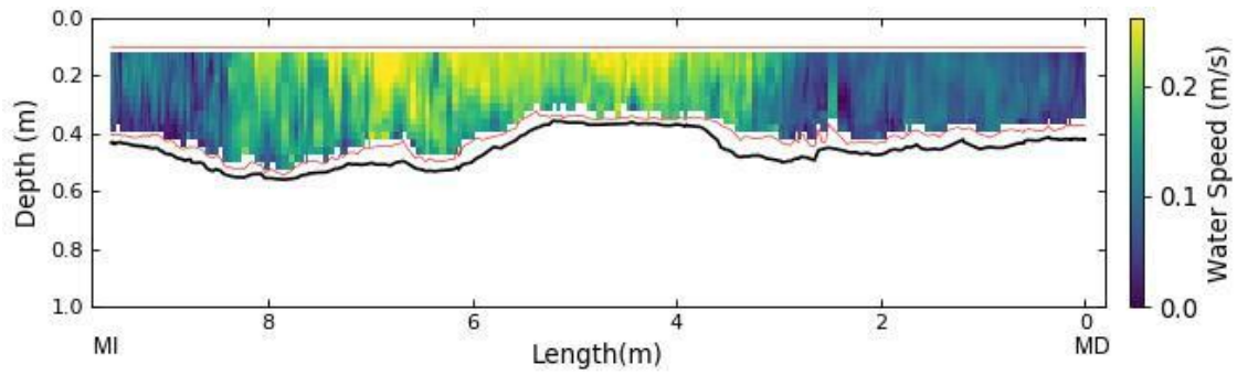
Figura A.10. Distribución de velocidades en la sección de aforo de la EM04 obtenida con ADCP. En el gráfico se señala la ubicación de la margen izquierda (MI) y de la margen derecha (MD).
