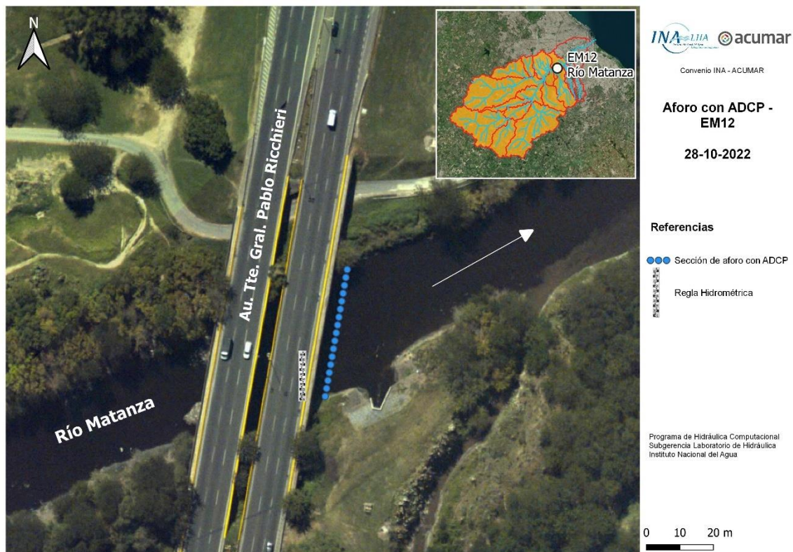
Figura A.25. Sección de aforo en la EM12.
