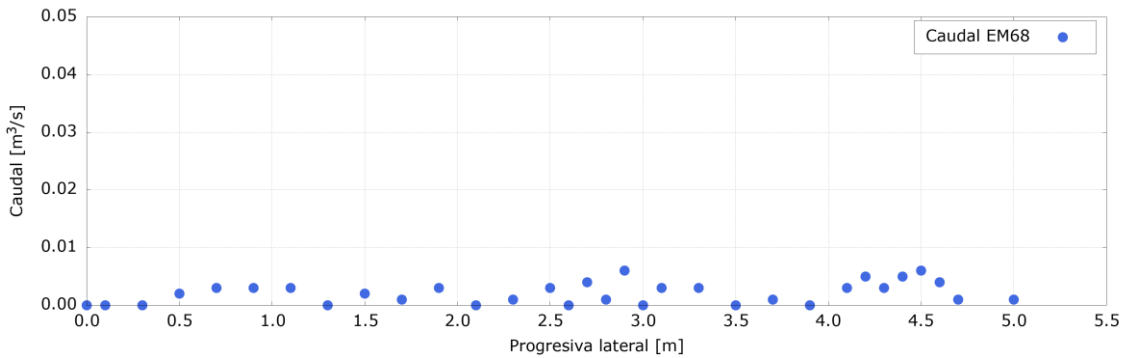
Figura A.80. Distribución de profundidades, velocidades medidas y caudales en la sección de aforo de la EM68 obtenida con ADV. La progresiva lateral 0 se corresponde con la margen izquierda.
