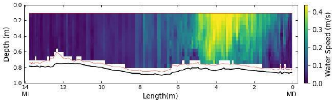
Figura A.23. Distribución de velocidades en la sección de aforo de la EM11 obtenida con ADCP. En el gráfico se señala la ubicación de la margen izquierda (MI) y de la margen derecha (MD).
