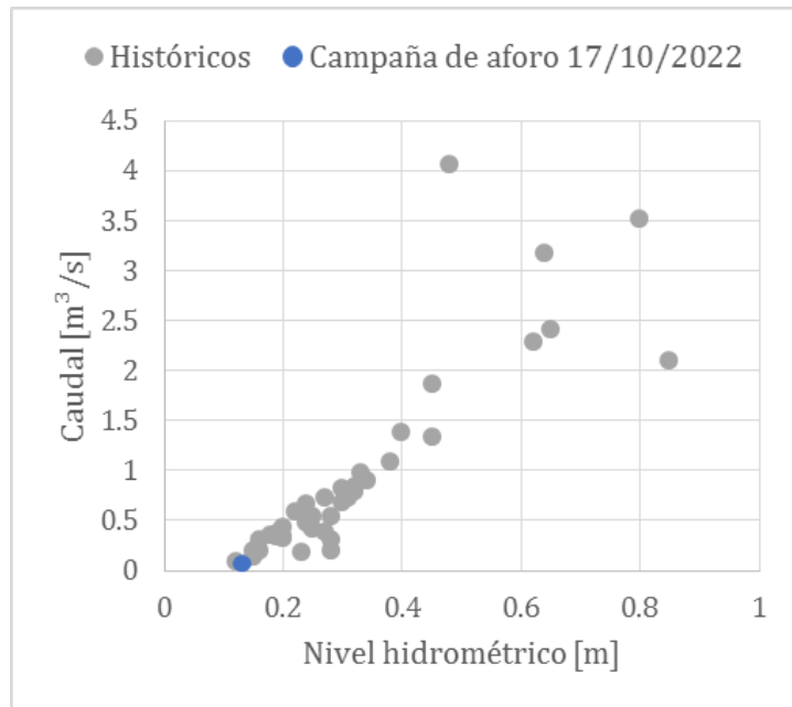
Figura A.81. Registros históricos de niveles y caudales en la EM68.
