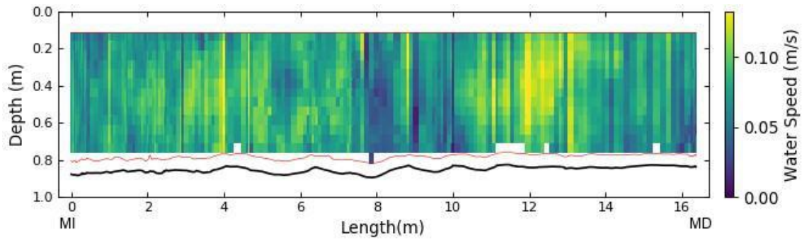
Figura A.100. Distribución de velocidades en la sección de aforo de la EM78 obtenida con ADCP. En el gráfico se señala la ubicación de la margen izquierda (MI) y de la margen derecha (MD).
