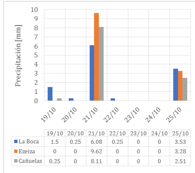
Figura A.93. Precipitaciones en la cuenca en la semana previa al aforo.
