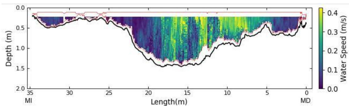
Figura A.29. Distribución de velocidades en la sección de aforo de la EM12 obtenida con ADCP. En el gráfico se señala la ubicación de la margen izquierda (MI) y de la margen derecha (MD).
