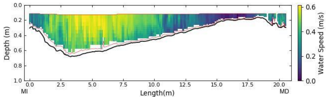
Figura A.34. Distribución de velocidades en la sección de aforo de la EM13 obtenida con ADCP. En el gráfico se señala la ubicación de la margen izquierda (MI) y de la margen derecha (MD).
