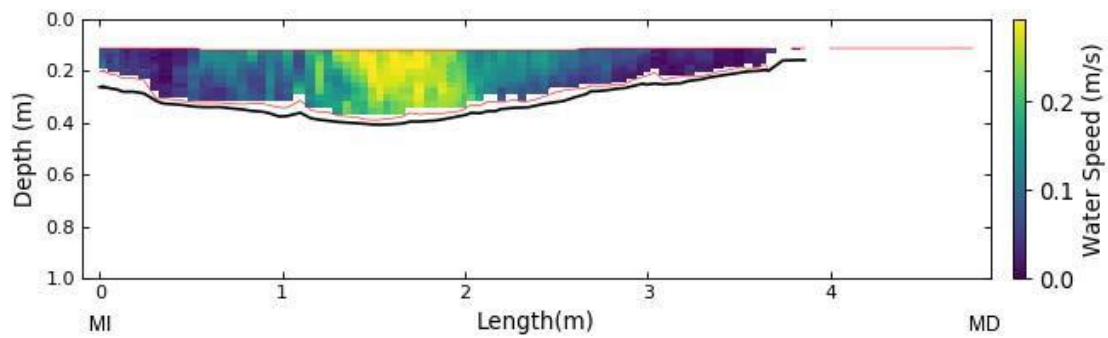
Figura A.5. Distribución de velocidades en la sección de aforo de la EM03 obtenida con ADCP. En el gráfico se señala la ubicación de la margen izquierda (MI) y de la margen derecha (MD).
