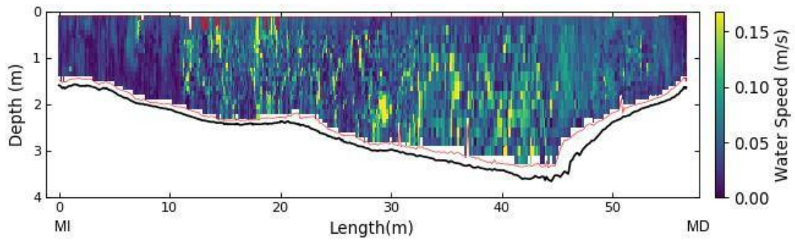
Figura A.54. Distribución de velocidades en la sección de aforo de la EM19 obtenida con ADCP. En el gráfico se señala la ubicación de la margen izquierda (MI) y de la margen derecha (MD).
