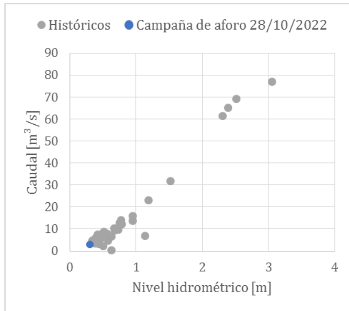
Figura A.30. Registros históricos de niveles y caudales en la EM12.
