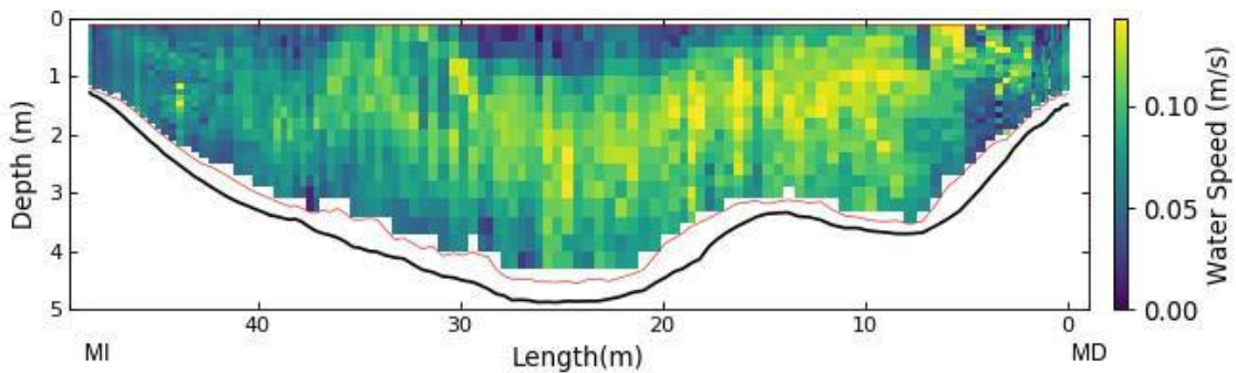
Figura A.65. Distribución de velocidades en la sección de aforo de la EM24 obtenida con ADCP. En el gráfico se señala la ubicación de la margen izquierda (MI) y de la margen derecha (MD).
