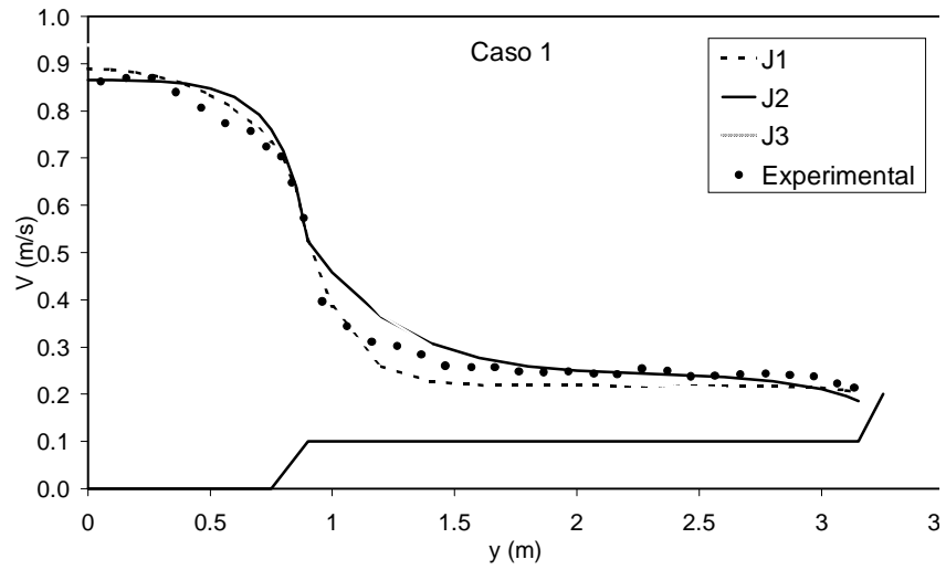
Figura 14.- Perfil de velocidades calculado con LDM – Caso 1
