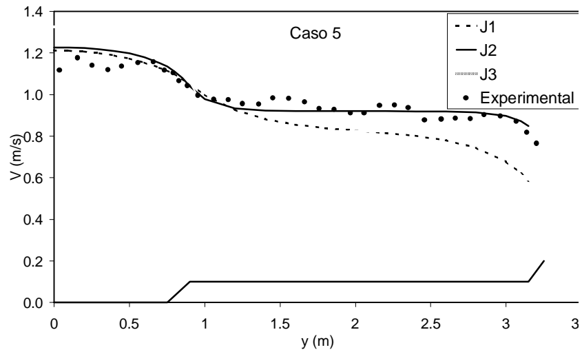
Figura 15.- Perfil de velocidades calculado con LDM – Caso 5
