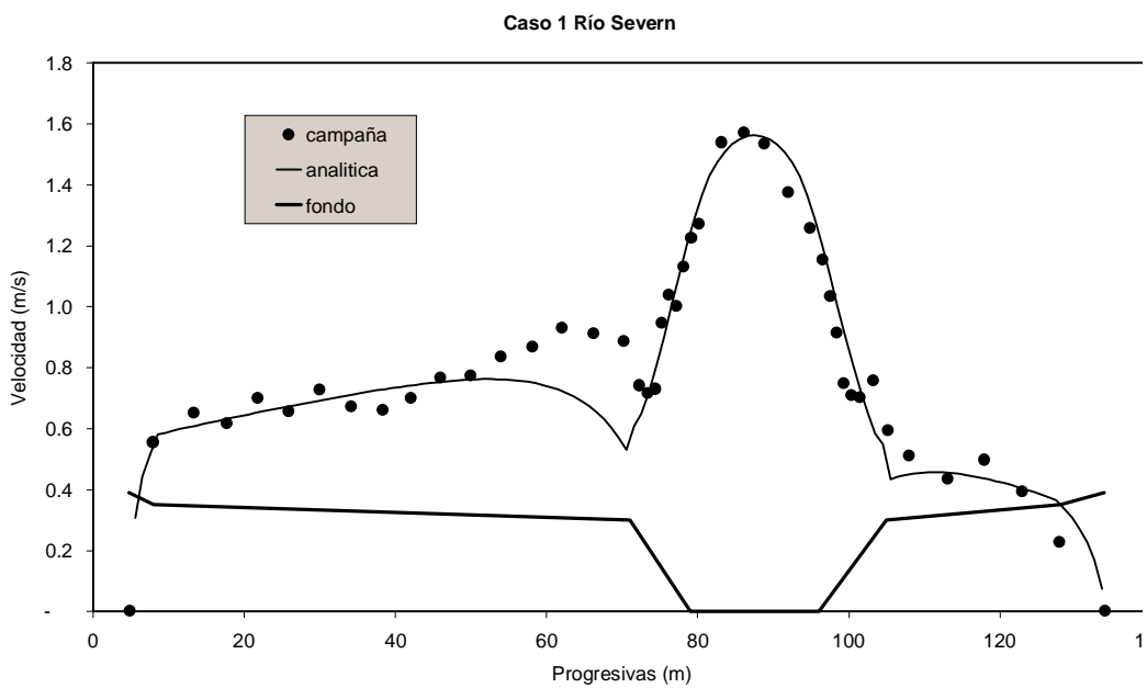
Figura 16.- Perfil de velocidades calculado con LDM – Caso 1
