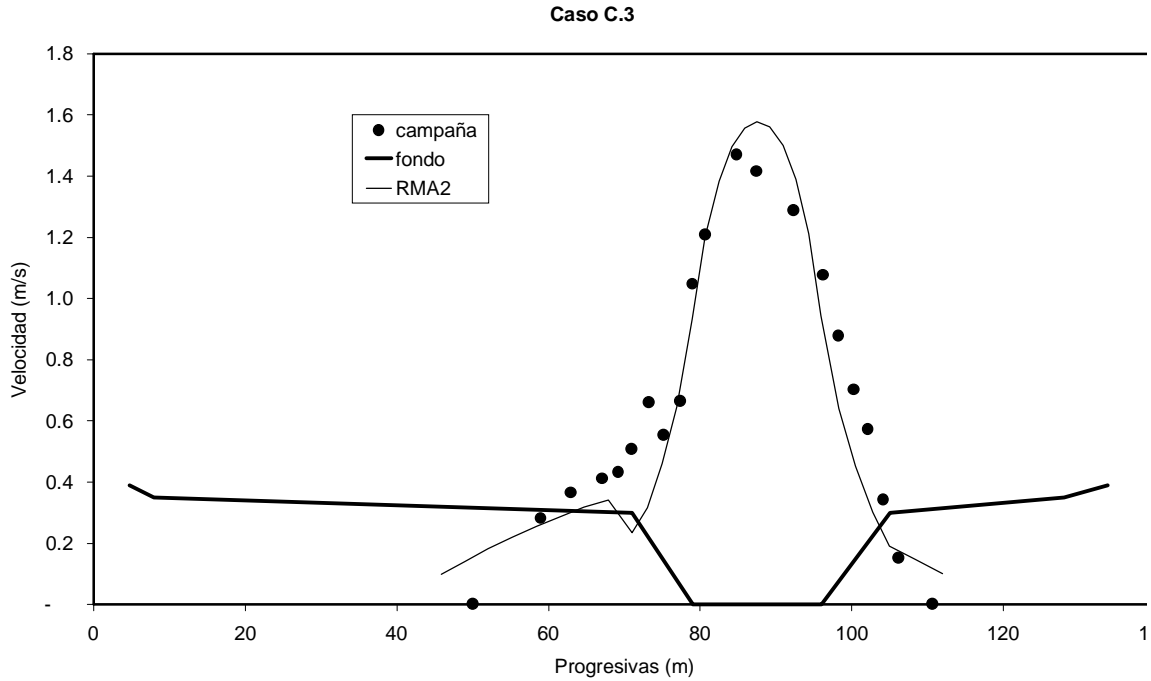
Figura 24.- Perfil lateral de velocidades calculado con RMA2 – caso 3 río Severn
