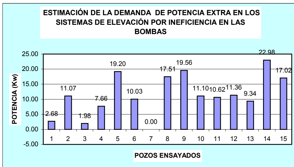
Figura 1. Demanda de potencia extra por ineficiencia en las bombas
